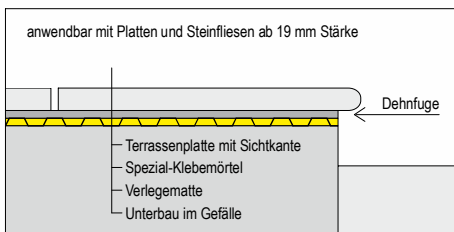
Verlegematte mit Spezial-Klebemörtel
