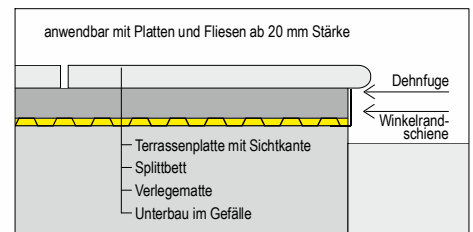
Verlegematte mit Splittbett
