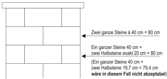
Pfeilerbreite 80 cm = zwei ganze Steine
