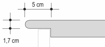
B Vario-Profil
