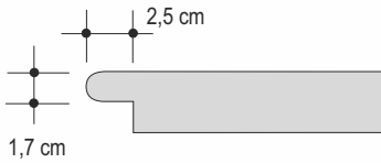
A Standard-Profil
